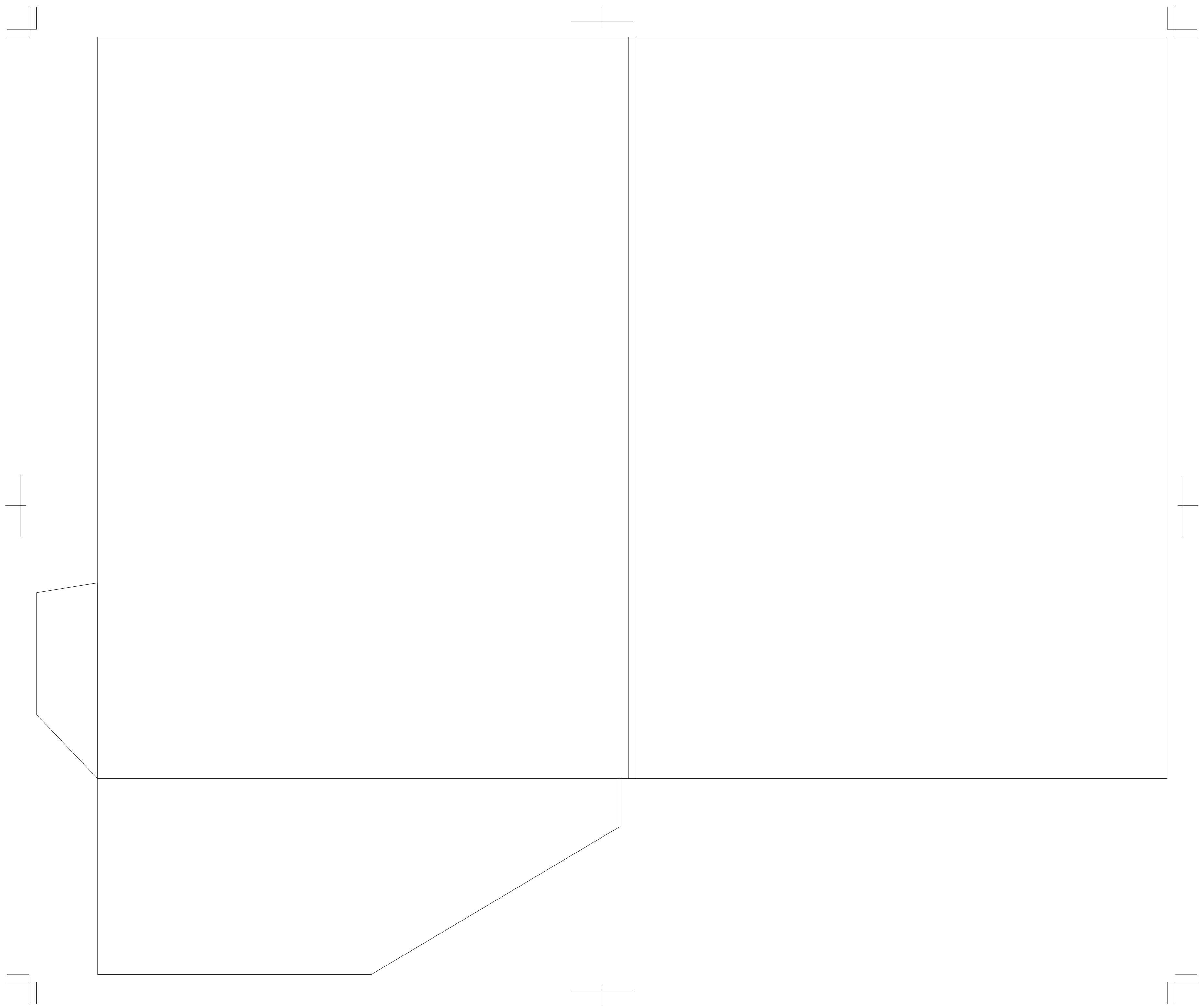
【片袖用】 外側印刷面展開図
